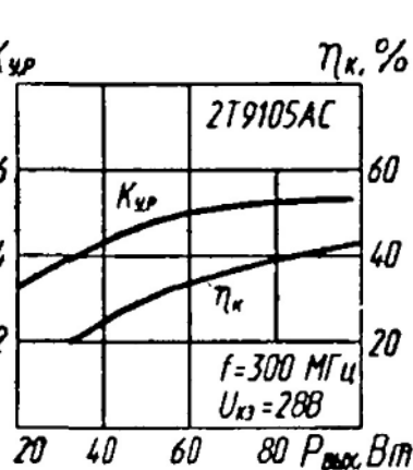
Зависимости коэффициента усиления и коэффициента полезного действия от выходной мощности
