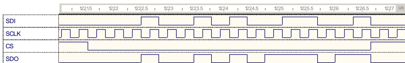
Рисунок 9 – Диаграмма записи по адресу 0x04 для микросхем третьей ревизии а) значения 0b10111011; б) значения 0b10011001.
