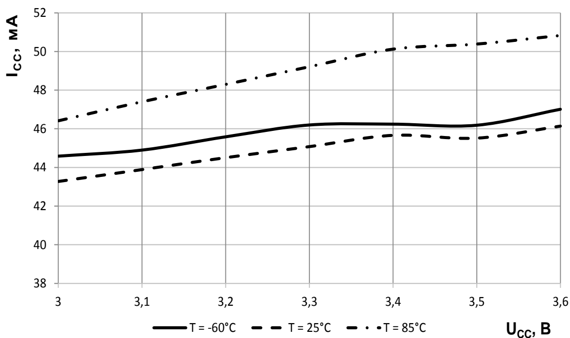
Рисунок 15 – Зависимость статического тока потребления от напряжения источника питания на выводах VDDA
