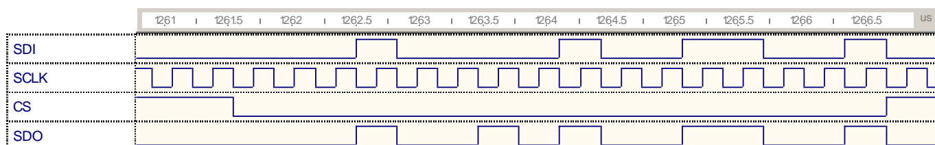
Рисунок 10 – Чтение из регистра по адресу 0x04 значения 0b10011001 для микросхем третьей ревизии
