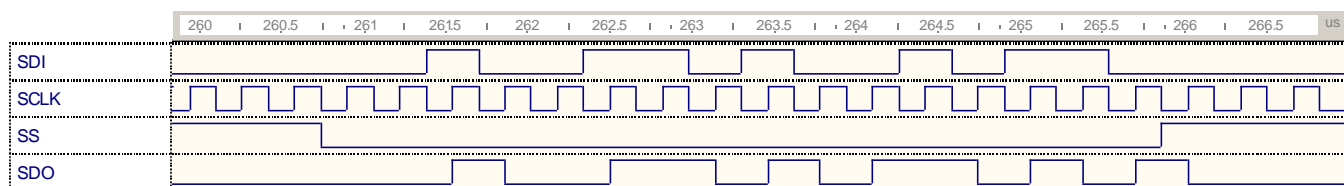
Рисунок 7 – Диаграмма записи по адресу 0x04 а) значения 0b10110101; б) значения 0b10010110.
