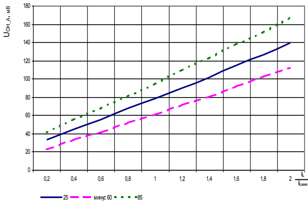
Рисунок 18 – Зависимость выходного напряжения высокого уровня аналоговых выходов txdp[3:0] , txdm[3:0] , dtror[3:0] , dtror[3:0] , xt2 , U_{OL\_A} , от тока нагрузки, при T=25\text{ }^{\circ}\text{C} , T=125\text{ }^{\circ}\text{C} , T=\text{минус } 60\text{ }^{\circ}\text{C} , |I_{Lnom}|=6\text{ mA}
