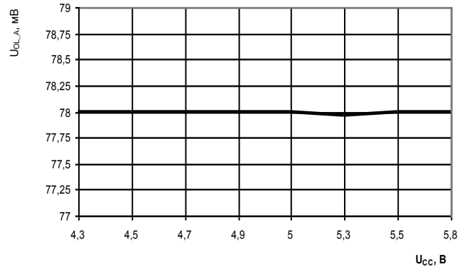
Рисунок 13 – Зависимость выходного напряжения низкого уровня аналоговых выходов txdp[3:0], txdm[3:0], dtrop[3:0], dtrom[3:0], xt2, U_{OL\_A} , от напряжения питания U_{CC} , при I_{OL}=6 \text{ мА} , T=25^\circ \text{С}
