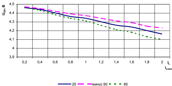
Рисунок 16 – Зависимость выходного напряжения высокого уровня цифровых выходов link_rec[3:0], partition[3:0], collision, chain_o, request_n, data_bus, U_{OH} , от изменения тока нагрузки, при T=25^\circ \text{С} , T=125^\circ \text{С} , T=\text{минус } 60^\circ \text{С} , |I_{Lnom}|=6 \text{ мА}
