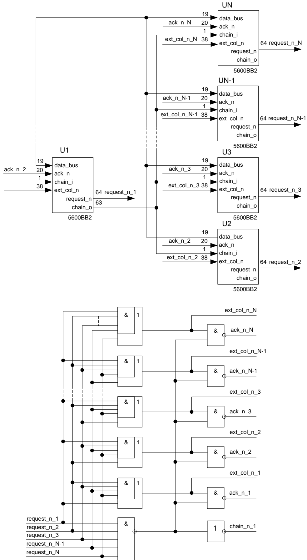
Рисунок 3 – Схема реализации устройства на базе двух и более микросхем, объединенных через порт расширения
