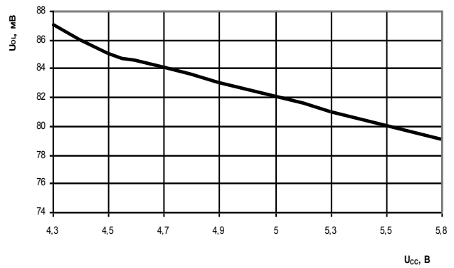
Рисунок 11 – Зависимость выходного напряжения низкого уровня цифровых выходов link_rec[3:0], partition[3:0], collision, chain_o, request_n, data_bus, U OL , от напряжения питания U cc , при I OL =6 мА, T=25°С
