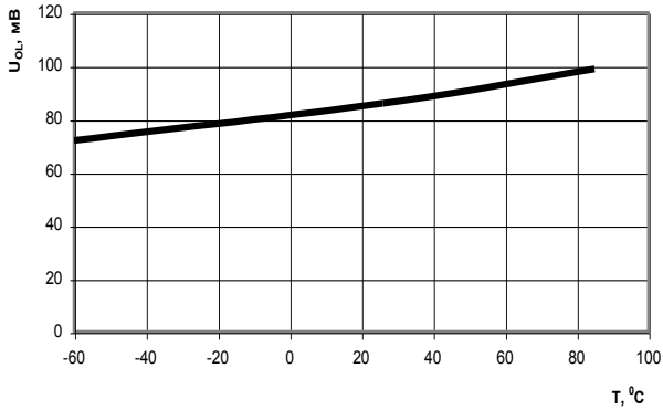
Рисунок 4 – Зависимость выходного напряжения низкого уровня цифровых выходов link_rec[3:0], partition[3:0], collision, chain_o, request_n, data_bus, U OL , от температуры Т°, при I OL =6 мА
