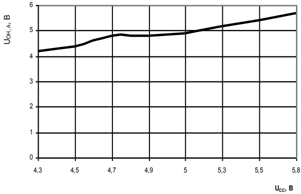
Рисунок 12 – Зависимость выходного напряжения высокого уровня аналоговых выходов txdp[3:0], txdm[3:0], dtrop[3:0], dtrom[3:0], xt2, U_{OH\_A} , от напряжения питания U_{CC} , при I_{OL}=\text{минус } 6 \text{ мА} , T=25^\circ \text{С} питания, при I_L=6 \text{ мА}
