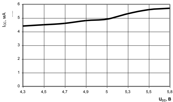
Рисунок 14 – Зависимость статического тока потребления I_{CC} от напряжения питания U_{CC} при T = 25^\circ \text{С}
