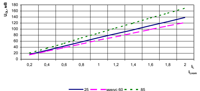
Рисунок 17 – Зависимость выходного напряжения низкого уровня цифровых выходов link_rec[3:0], partition[3:0], collision, chain_o, request_n, data_bus, U_{OL} , от тока нагрузки, при T=25^\circ \text{С} , T=125^\circ \text{С} , T=\text{минус } 60^\circ \text{С} , |I_{Lnom}|=6 \text{ мА}
