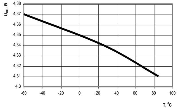
Рисунок 5 – Зависимость выходного напряжения высокого уровня цифровых выходов link_rec[3:0], partition[3:0], collision, chain_o, request_n, data_bus, U OH , от температуры Т°, при I OL =минус 6 мА
