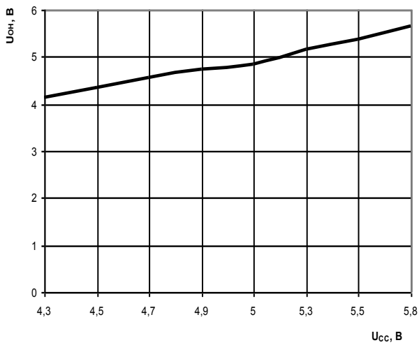
Рисунок 10 – Зависимость выходного напряжения высокого уровня цифровых выходов link_rec[3:0], partition[3:0], collision, chain_o, request_n, data_bus, U OH , от напряжения питания U cc , при I OL =минус 6 мА, T=25°С
