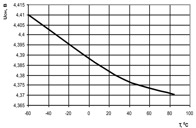
Рисунок 7 – Зависимость выходного напряжения высокого уровня аналоговых выходов txdp[3:0], txdm[3:0], dtpop[3:0], dtpom[3:0], xt2, U OH_A , от температуры Т°, при I OL =минус 6 мА
