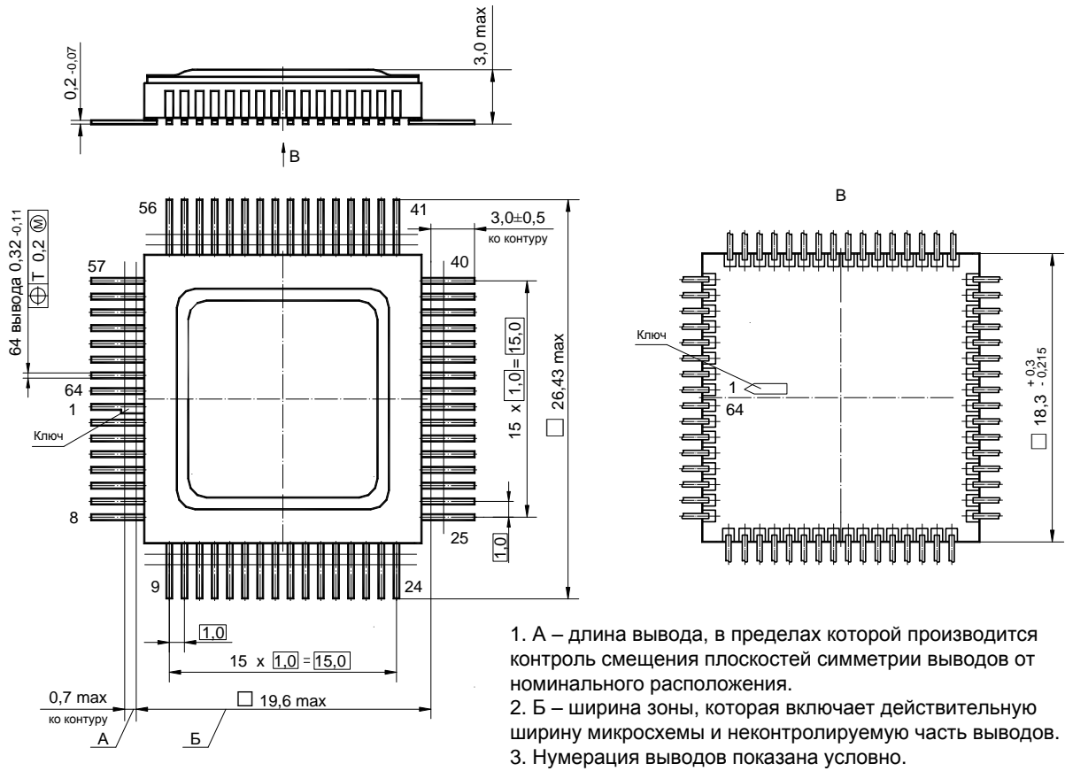
Рисунок 20 – Микросхема в корпусе N18.64-1B
