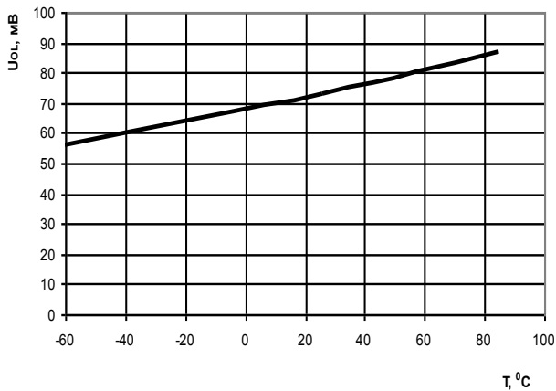
Рисунок 6 – Зависимость выходного напряжения низкого уровня аналоговых выходов txdp[3:0], txdm[3:0], dtpop[3:0], dtpom[3:0], xt2, U OL_A , от температуры Т°, при I OL =6 мА
