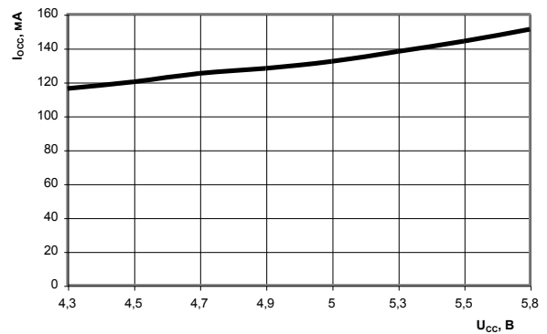
Рисунок 15 – Зависимость динамического тока потребления I_{OCC} от напряжения питания U_{CC} при T = 25^\circ \text{С}
