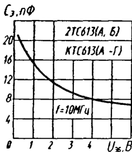
Зависимость емкости эмиттерного перехода от напряжения эмиттер—база
