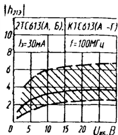
Зона возможных положений зависимости модуля коэффициента передачи тока от напряжения коллектор—база
