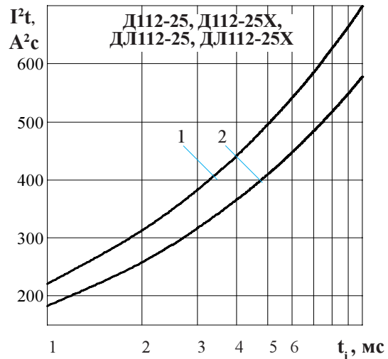
Рисунок 9 - Зависимость защитного показателя \Gamma^2t от длительности импульса тока t_i при исходной температуре структуры T_j = 25 C (1) и максимальной температуре T_{jm} (2)
