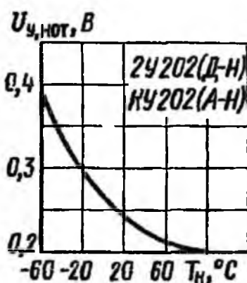
Зависимость неотпирающего постоянного напряжения управления от температуры корпуса
