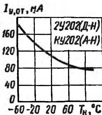
Зависимость отпирающего постоянного тока управления от температуры корпуса
