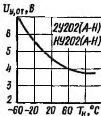
Зависимость отпирающего постоянного напряжения управления от температуры корпуса
