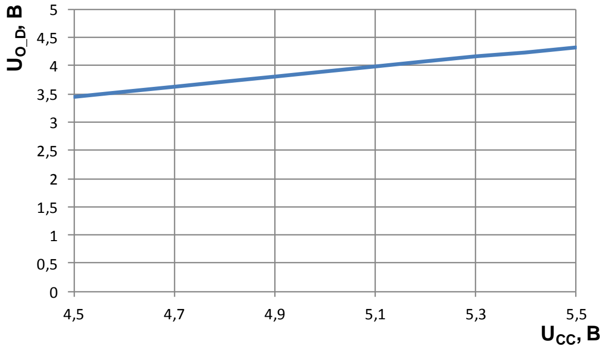
Рисунок 6 – Зависимость выходного дифференциального напряжения передатчика U_{o\_D} от напряжения источника питания при T=25\text{ }^{\circ}\text{C}
