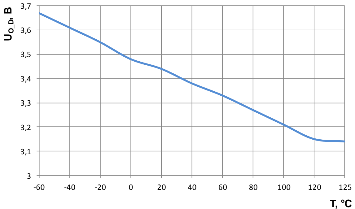
Рисунок 7 – Зависимость выходного дифференциального напряжения передатчика U_{o\_D} от температуры при U_{CC} = 4,5\text{ В}
