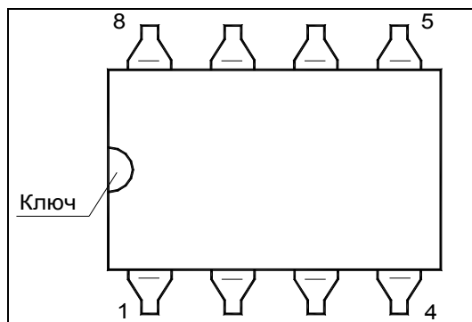
Схема расположения выводов
