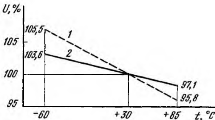
Рис 27 График изменения напряжения вторичных обмоток трансформаторов в режиме номинальной нагрузки в зависимости от температуры окружающей среды 1 — наименьший уход напряжения от значения, измеренного при нормальной температуре 2 — средний уход напряжения от значения, измеренного при нормальной температуре
