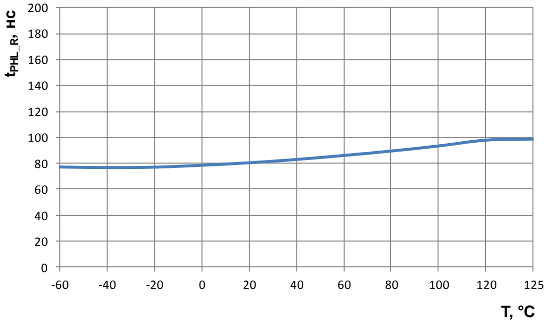
Рисунок 11 – Зависимость времени задержки распространения сигнала приемника при включении t_{PHL\_R} от температуры при U_{CC} = 4,5 В
