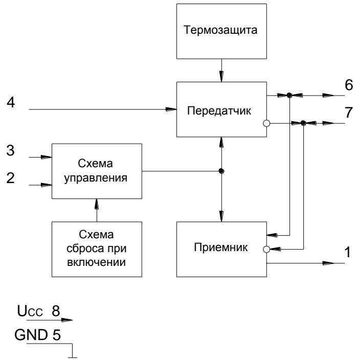
Рисунок 1 – Структурная блок-схема микросхемы
