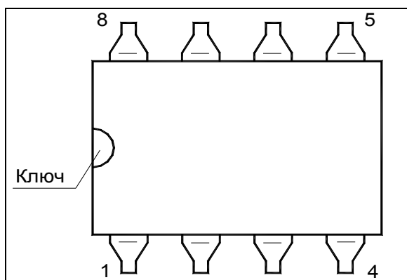
Схема расположения выводов
