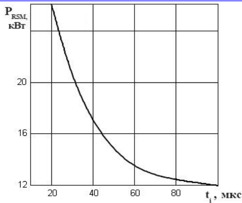
Рисунок 12: Зависимость допустимой ударной обратной рассеиваемой мощности P_{RSM} от длительности одиночного импульса t_1 обратного тока синусоидальной формы в состоянии лавинного пробоя при максимальной температуре структуры T_{jm} .
