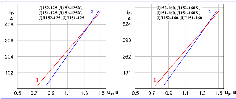
Рисунок 1: Пределные вольтамперные характеристики при максимально допустимой температуре перехода T_{jm} (1) и температуре T_j=25^\circ\text{C} (2), I_F=3,14 I_{F(AV)} .
