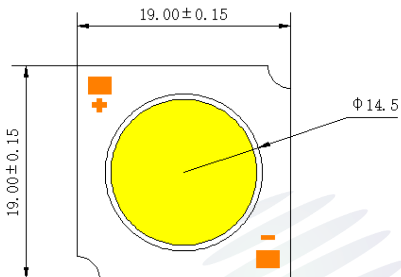
Fig.1-1 Top view 正面视图
