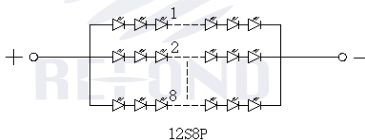
Fig.1-3 Polarity 极性
